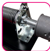
Option ressort de torsion. Syst-ème «parachute» : interdit la chute du tablier en cas de défaillance du ressort
